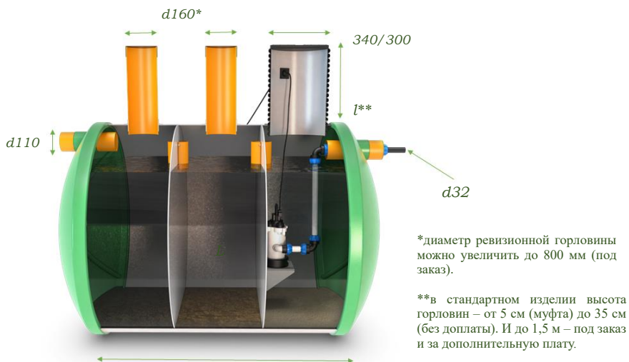
Рис 1. Устройство септика
